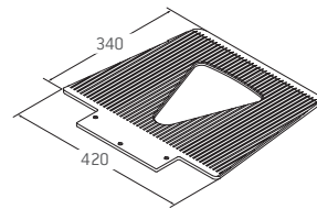
Schaufel G (420x340x7 mm) für große Pakete MAPO Art.-Nr. E/1543.930003
