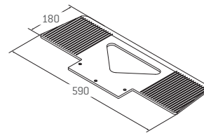
Schaufel XLW (590x180x7 mm) auch für Weißgut, Füße stehen auf Schaufel MAPO Art.-Nr. E/1543.930074
