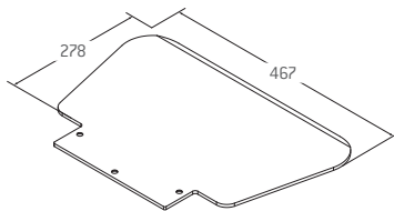
Schaufel LH (467x278x5 mm) wie Schaufel V, jedoch größer MAPO Art.-Nr. E/1543.930002
