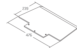
Schaufel GS-NG (476x239x7 mm) für Kartonware (z.B.: Getränkedosen) MAPO Art.-Nr. E/1543.930084
