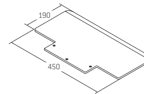
Schaufel DS-NG (450x190x7 mm) auch für Kartonwaren MAPO Art.-Nr. E/1543.930085
