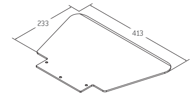
Schaufel V (413x233x5 mm) zum Transport von Sauerstoffbehältern MAPO Art.-Nr. E/1543.930001
