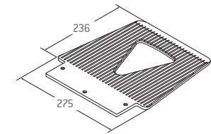
Schaufel Standard (275x236x7 mm) mit Längsrippen gegen seitliches Verrutschen MAPO Art.-Nr. E/1543.030025
